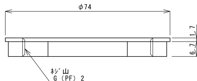
⑥ 締付ナット
