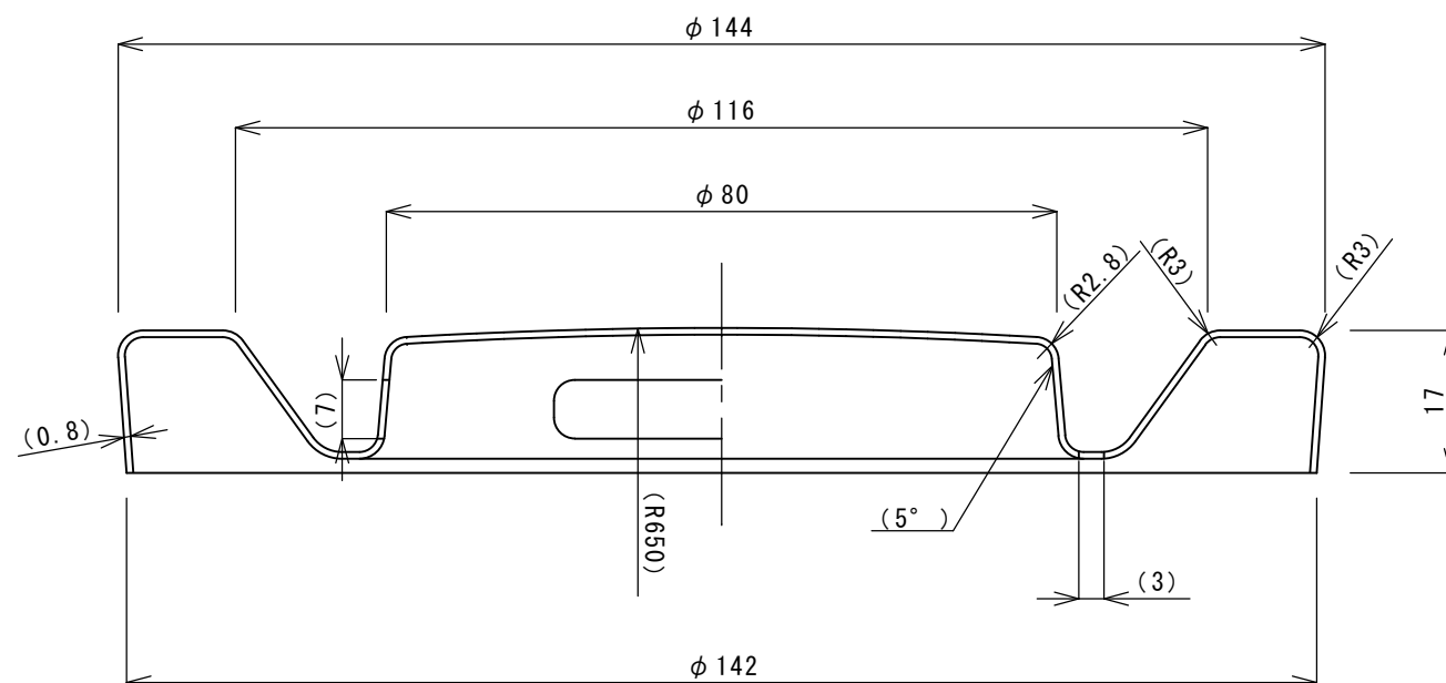
A-A' 断面
