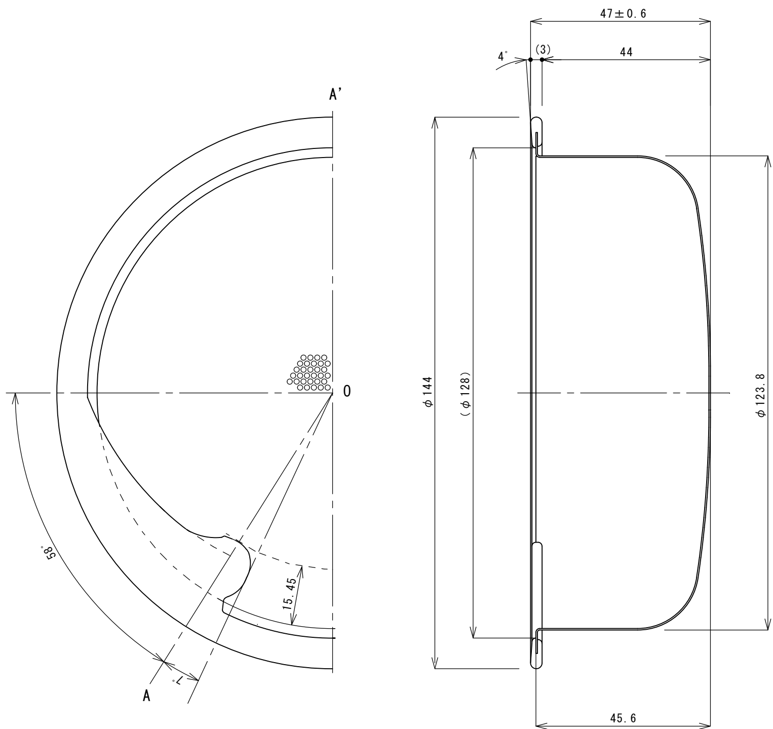
A-O-A' 断面
