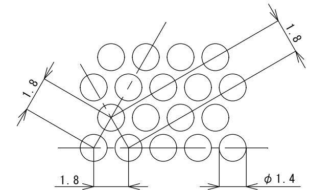
パンチング詳細 (5/1)
