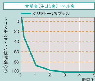
■トリメチルアミン消臭試験(社内試験)※1
