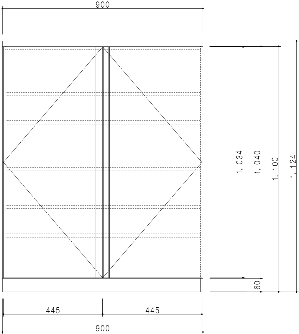
立面図
