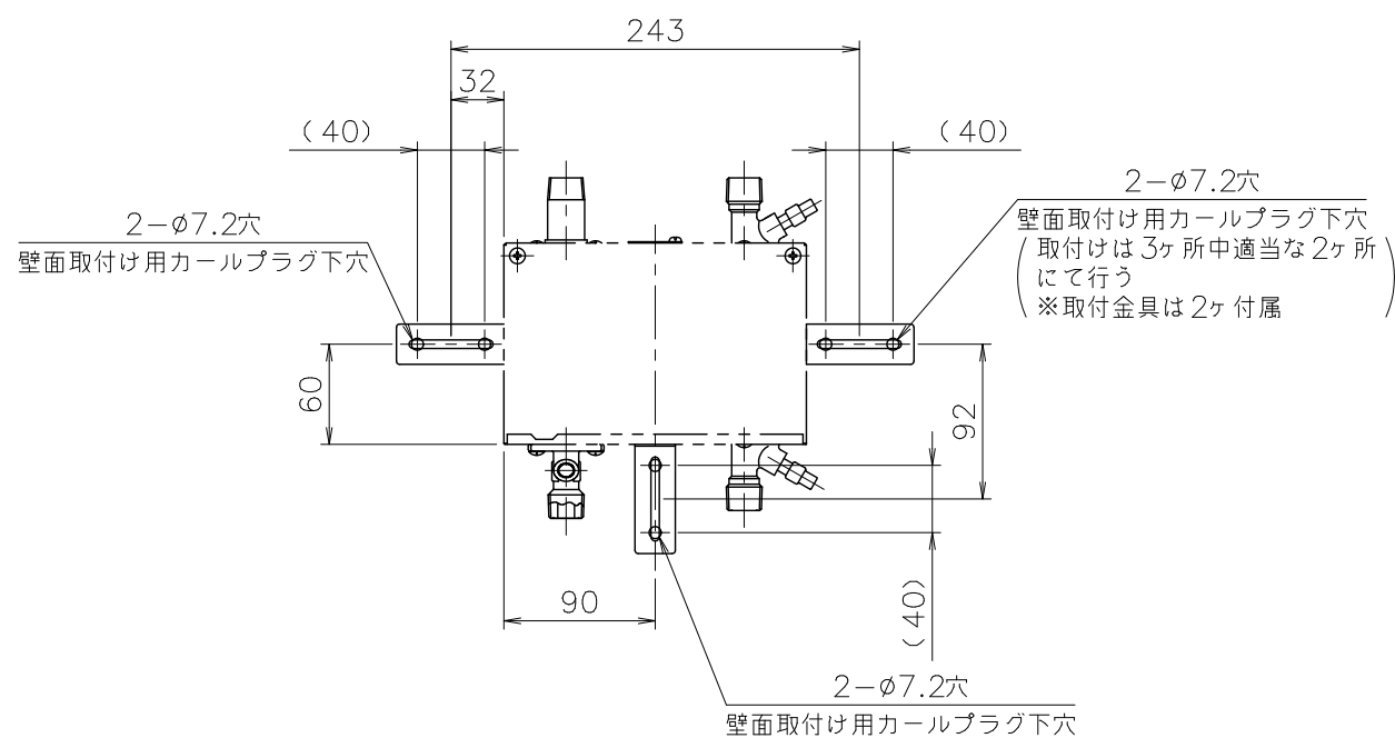
■取付参考図
