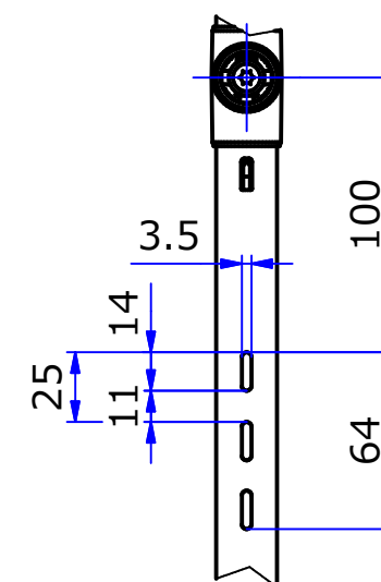
B ( 1 : 3 )
