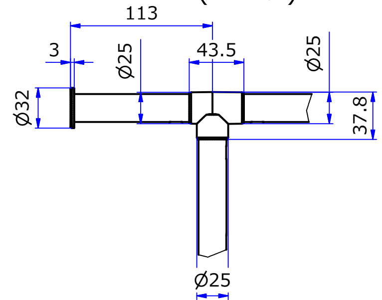
C ( 1 : 3 )
