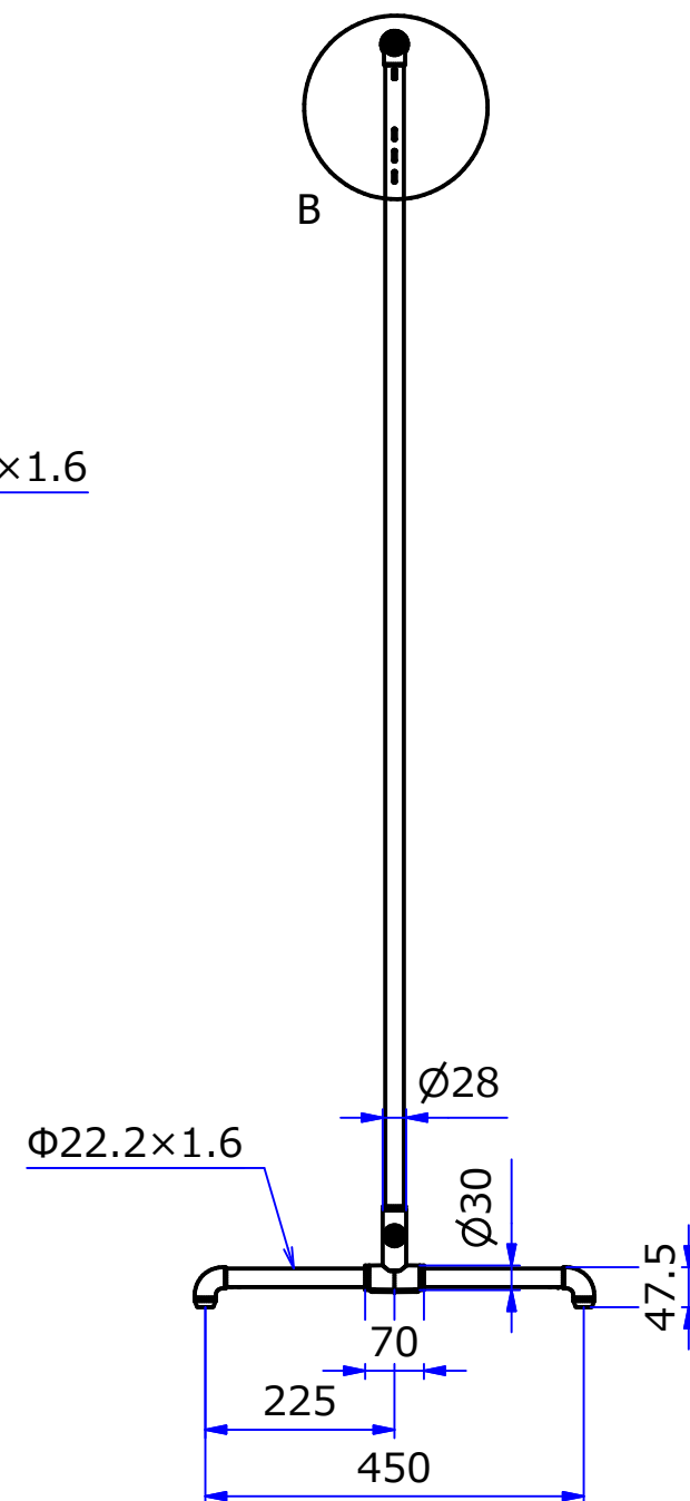
A-A ( 1 : 10 )
