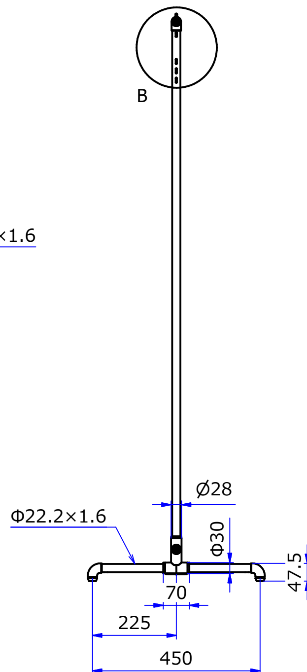
A-A ( 1 : 10 )
