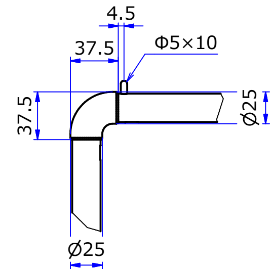
C ( 1 : 3 )
