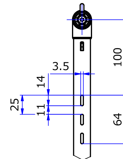
B ( 1 : 3 )
