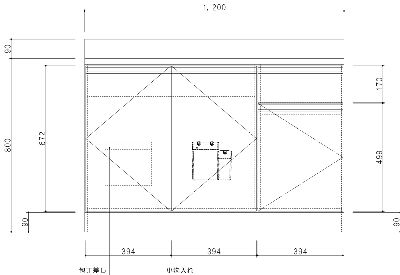
立面図
