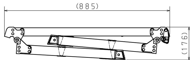
収納状態図
