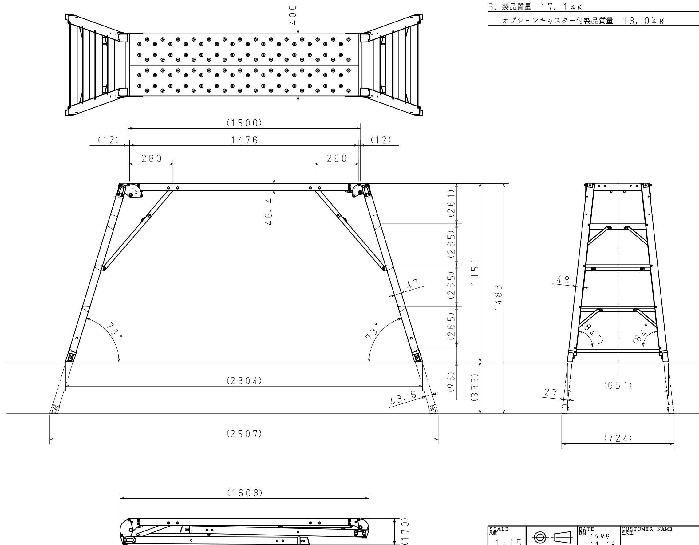
収納状態図
