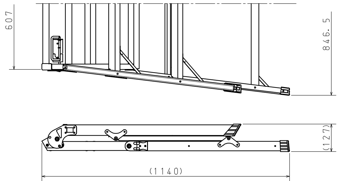
収納状態図
