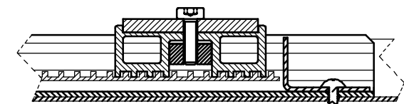
A-A断面図 (S = 1 : 2)
