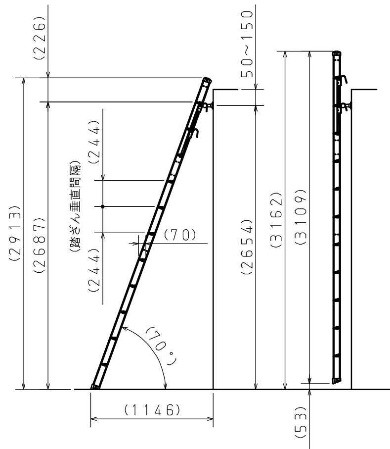
最大設置時 (S = 1 : 35)
