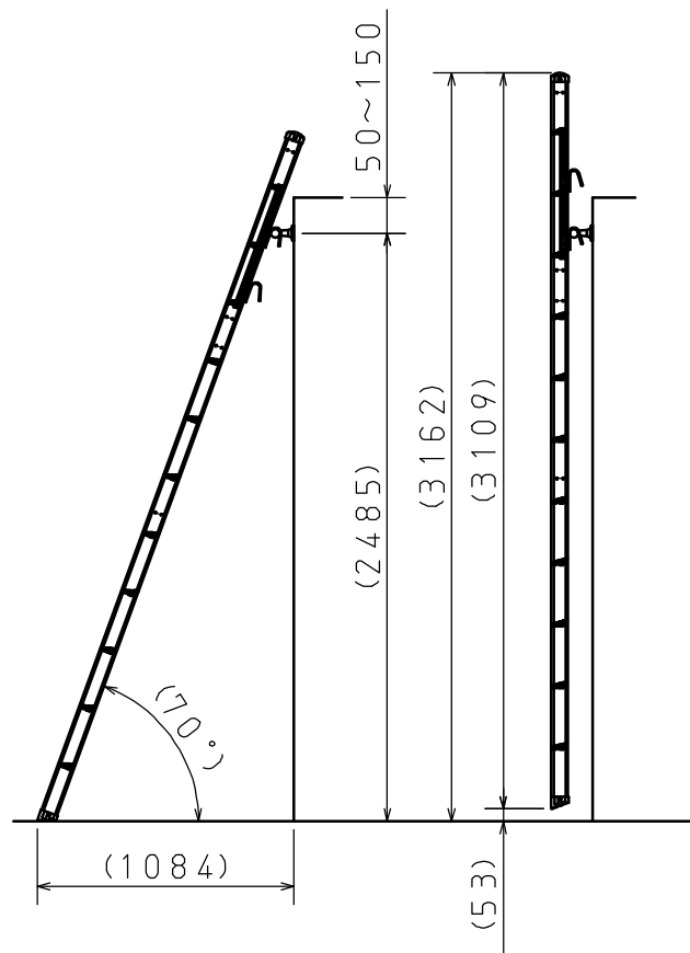
最小設置時 (S = 1 : 35)
