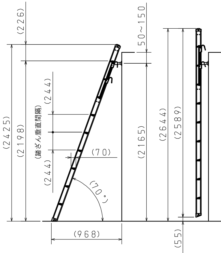
最大設置時 (S = 1 : 30)
