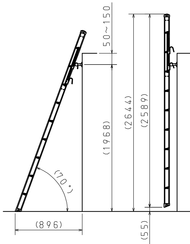
最小設置時 (S = 1 : 30)
