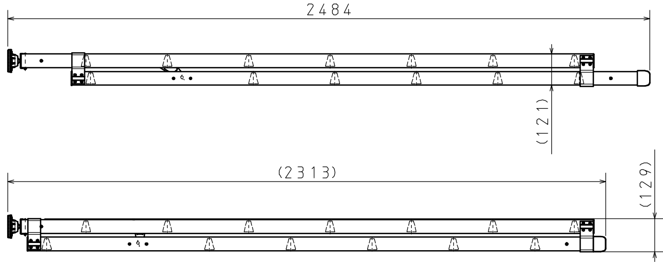
収納状態図
