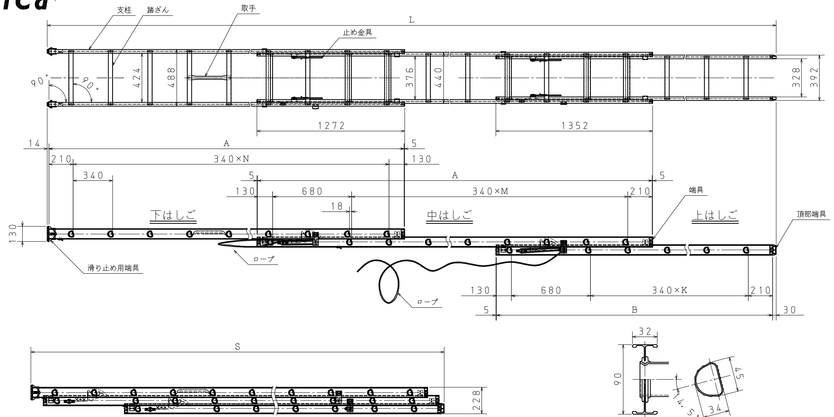
支柱・踏ざん詳細 (S=1:3)
