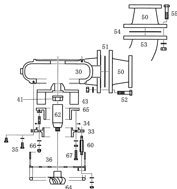
図-8 分解図 (立型)
