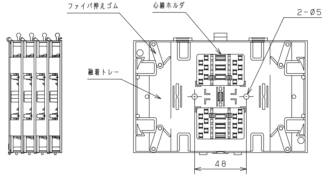
トレー内部詳細図
