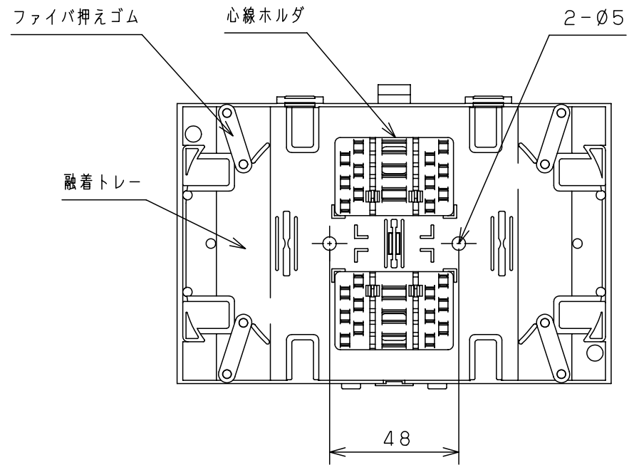
トレー内部詳細図
