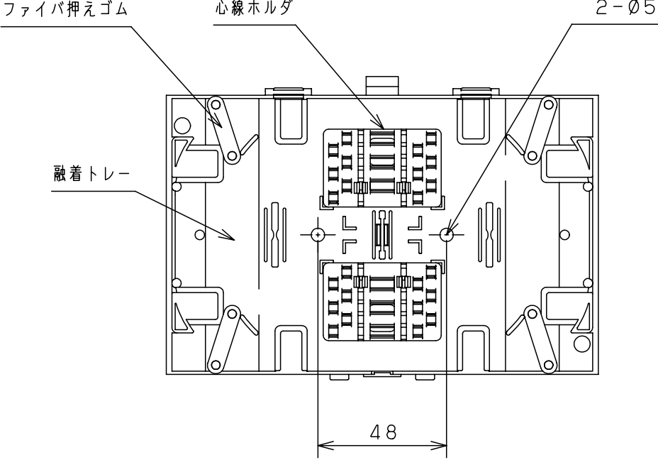
トレー内部詳細図
