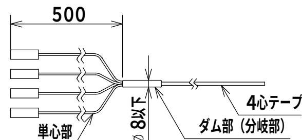
片端光コネクタ付FOコード推奨寸法
