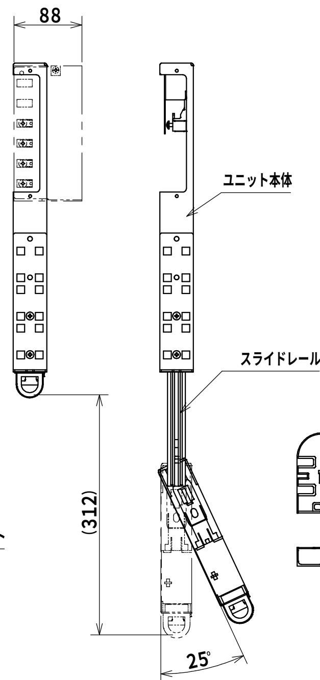
クランプユニット部 (1:3)
