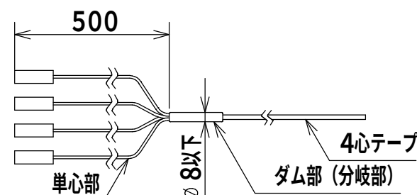
片端光コネクタ付F0コード推奨寸法
