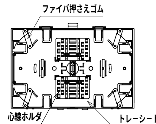
リール台2U (1:5)
