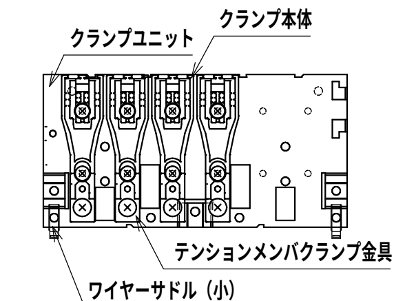
クランプユニット部 (1:3)
