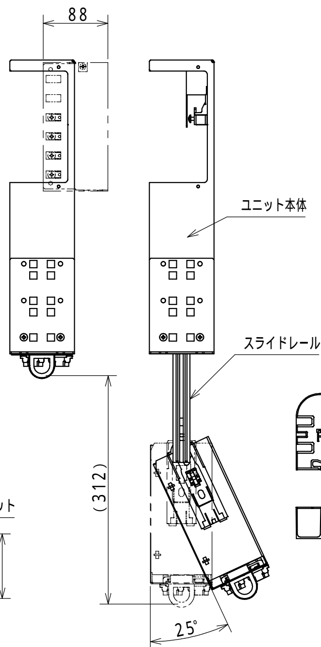
リール台2U (1:5)
