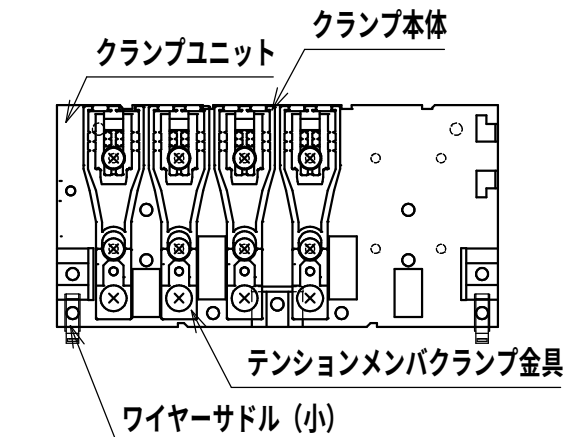
クランプユニット部 (1:3)
