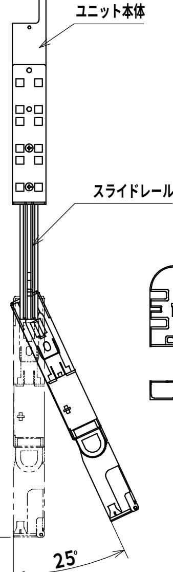
クランプユニット部 (1:3)
