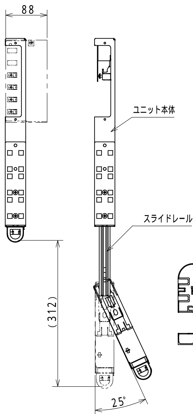
リール台1U (1:5)
