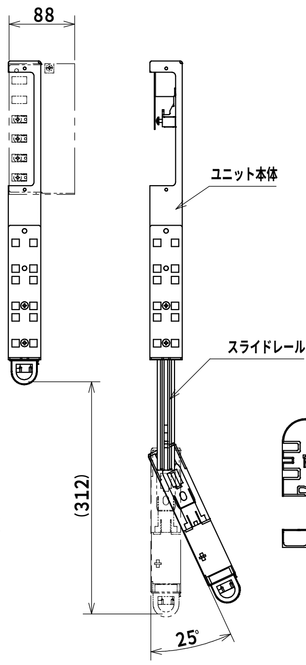
クランプユニット部 (1:3)
