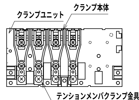
クランプユニット部 (1:3)
