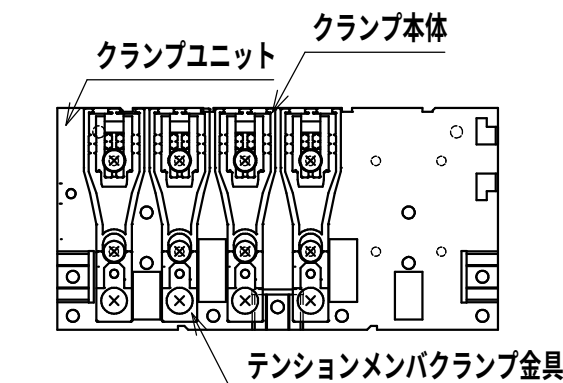
クランプユニット部 (1:3)
