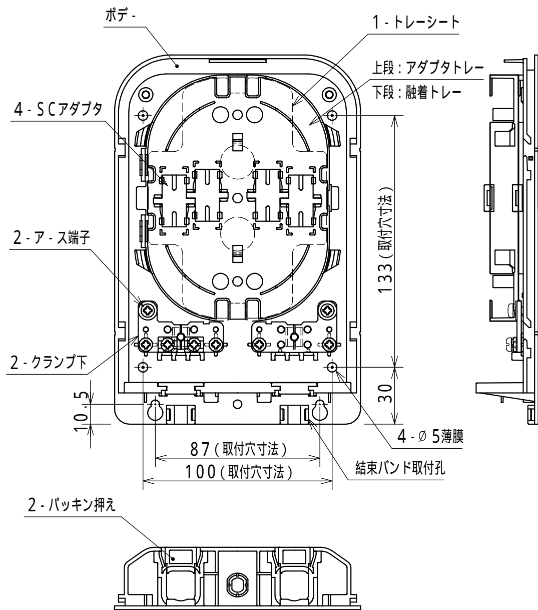
内部詳細図
