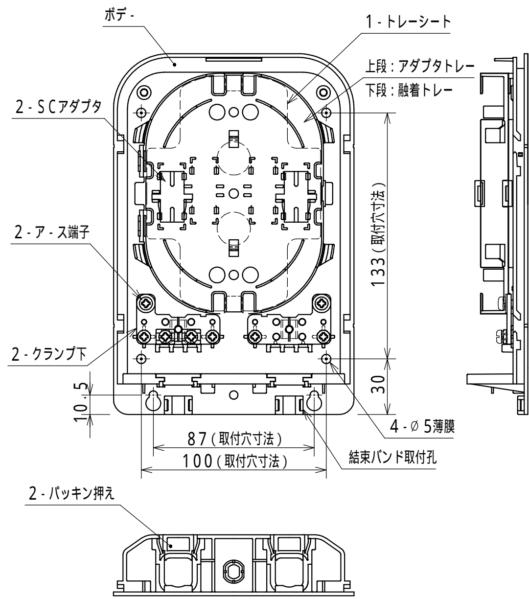
内部詳細図
