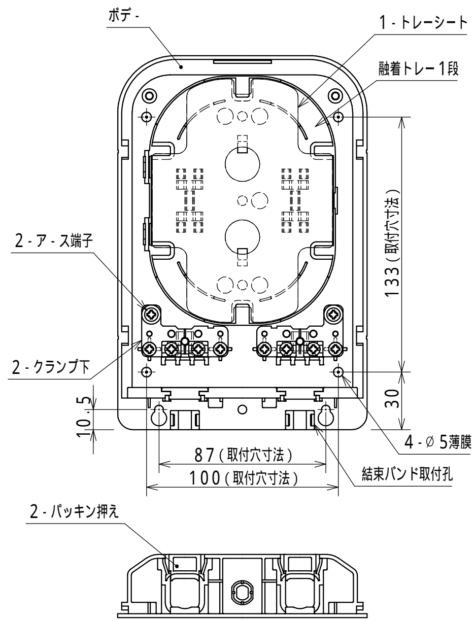
内部詳細図
