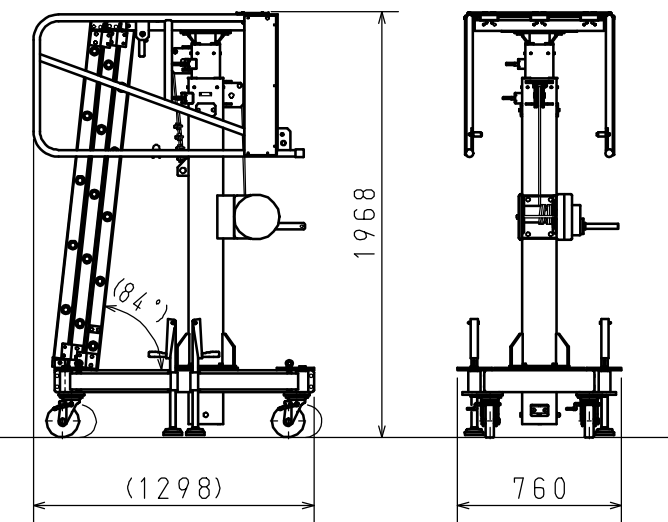
收納狀態
