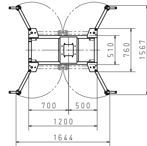
A-A矢視
