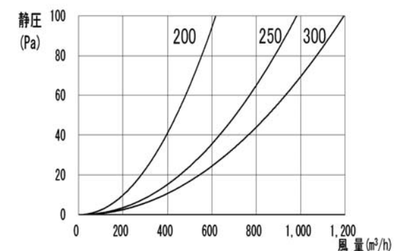
圧力損失曲線
