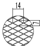
ワジョン ラス網 7×14 (呼称・5メッシュ)
