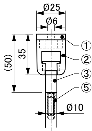
【B部 分解詳細(1:2)】
