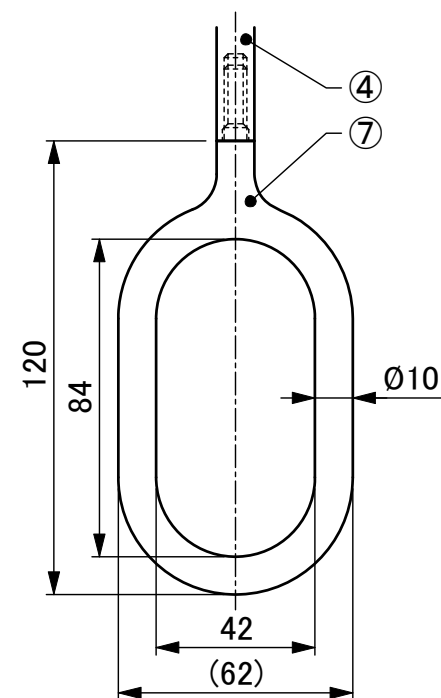
【C部 詳細(1:2)】
