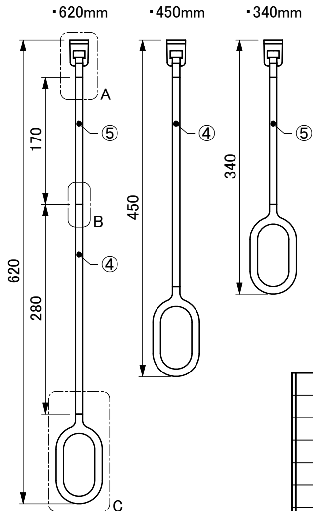
【高さ調整(3段階)】
