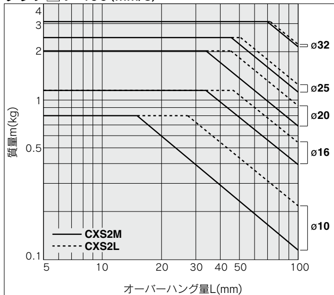
グラフ 8 V=700 (mm/s) (φ10はV=800)
