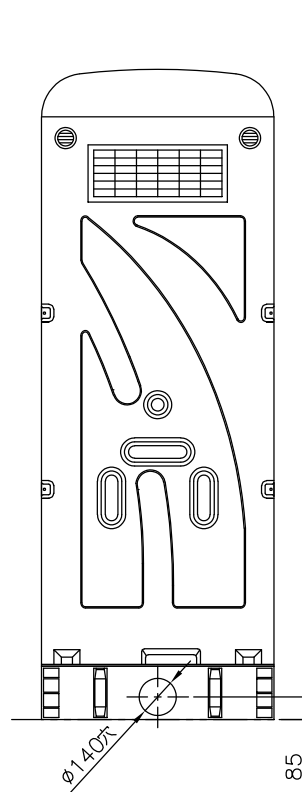
15WS架台伏せ図
