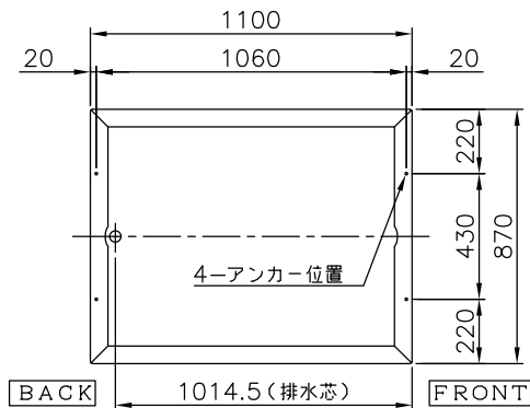
15WS架台伏せ図
