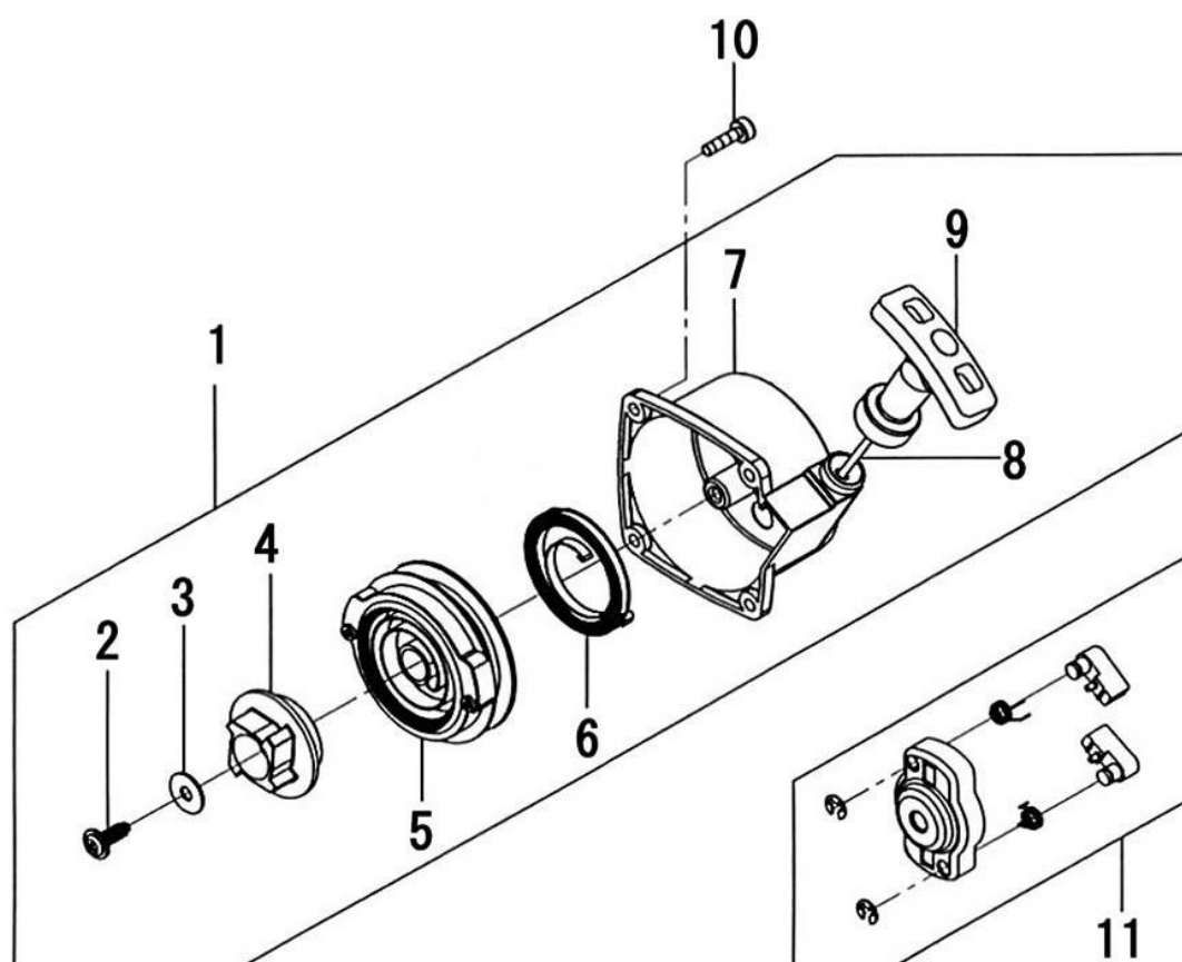
第7図 リコイルスターター部
