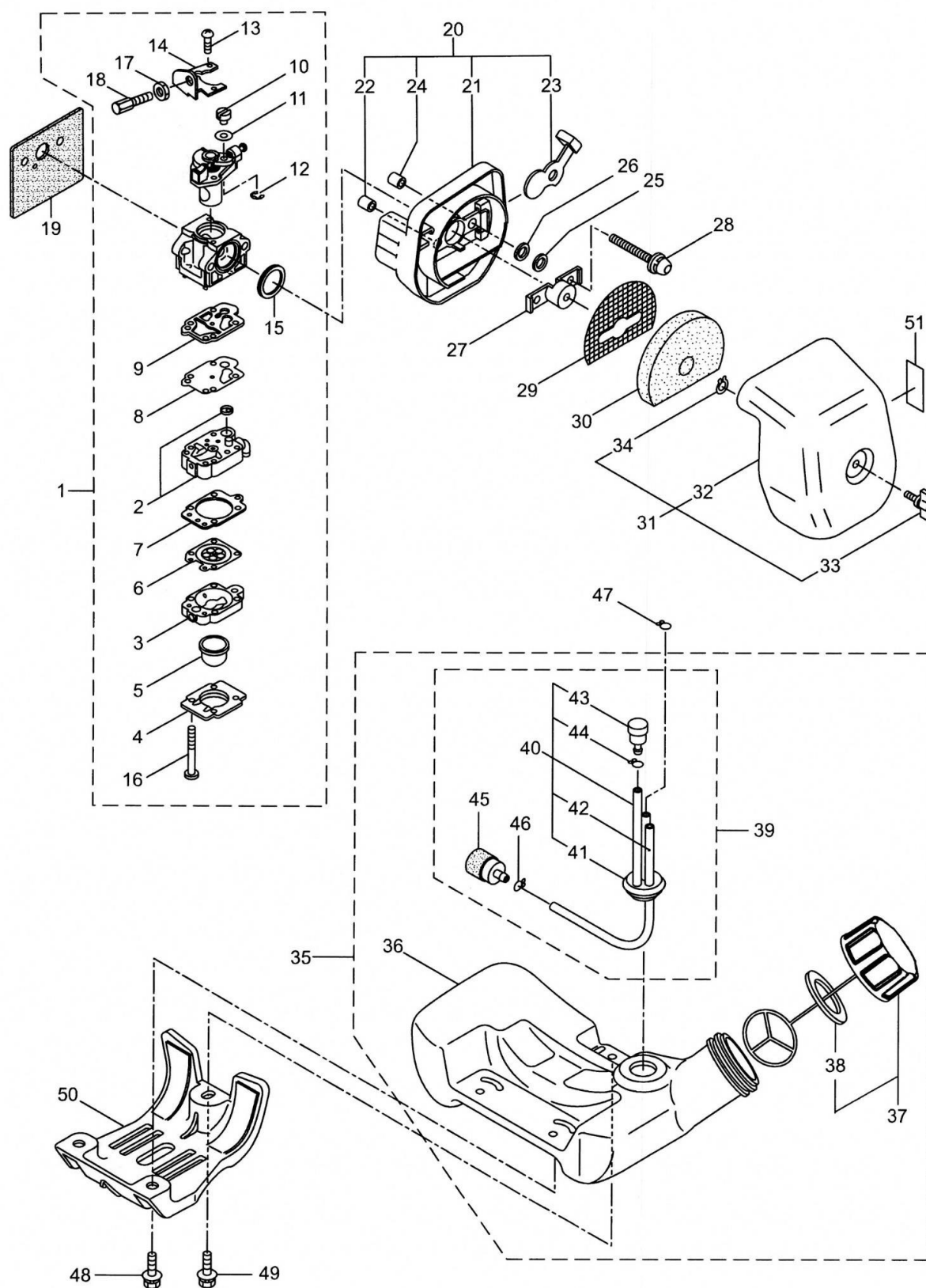
第3図 キャブレター/タンク部
