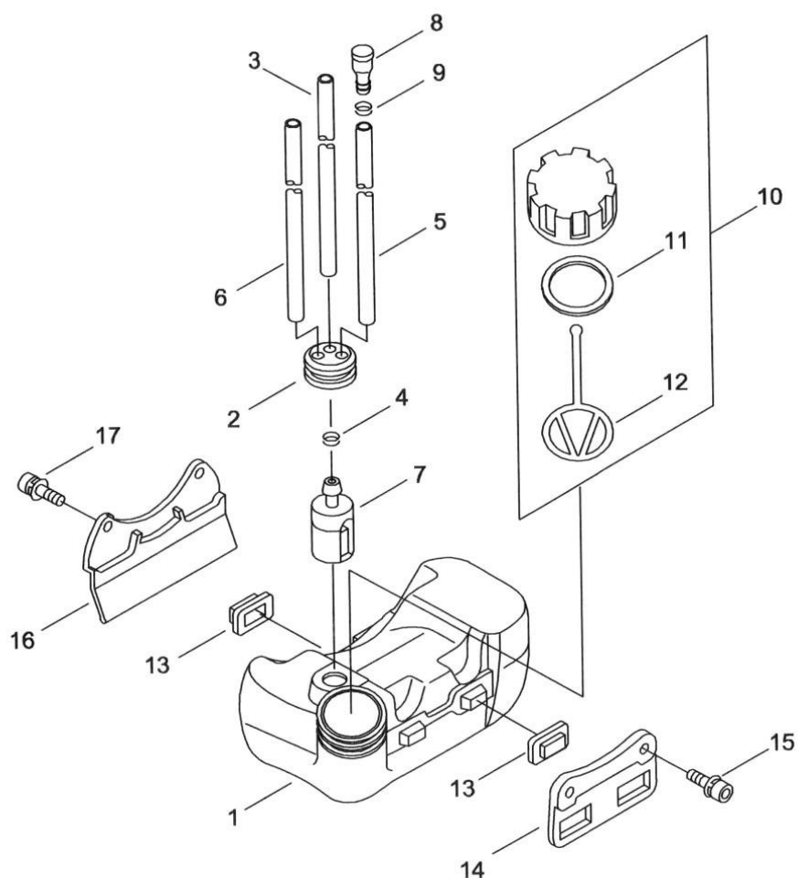
第6図 燃料タンク部
