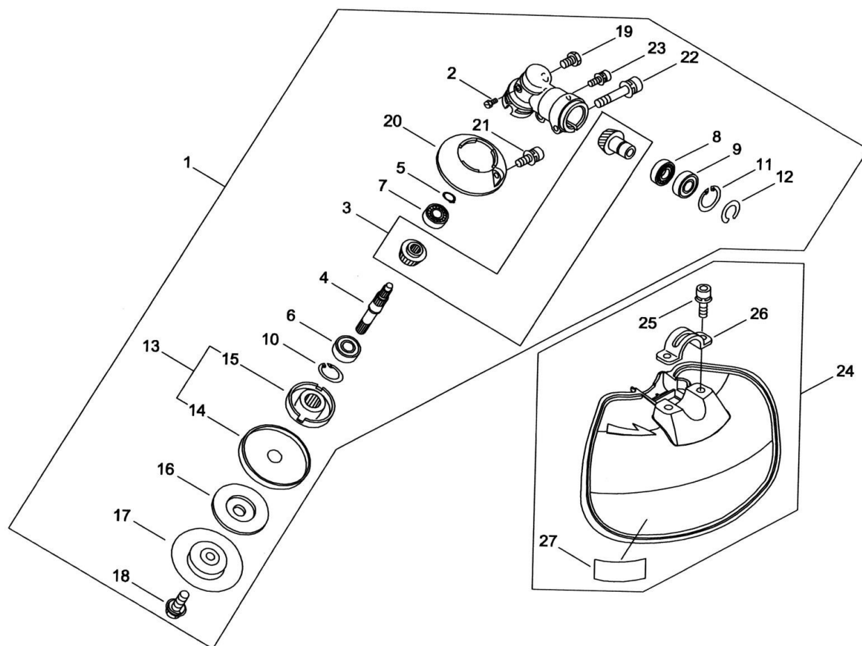
第11図 ギア部
