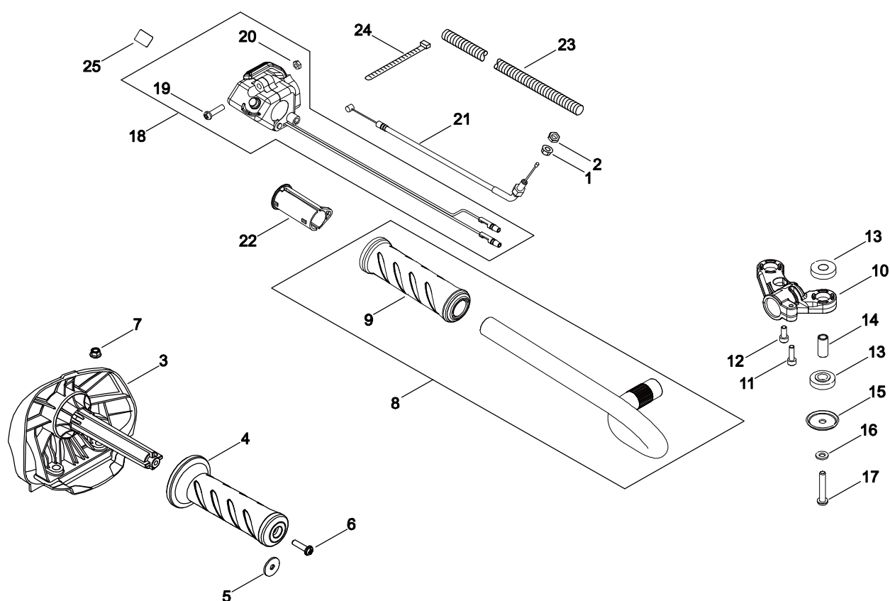
第11図 ハンドル部
