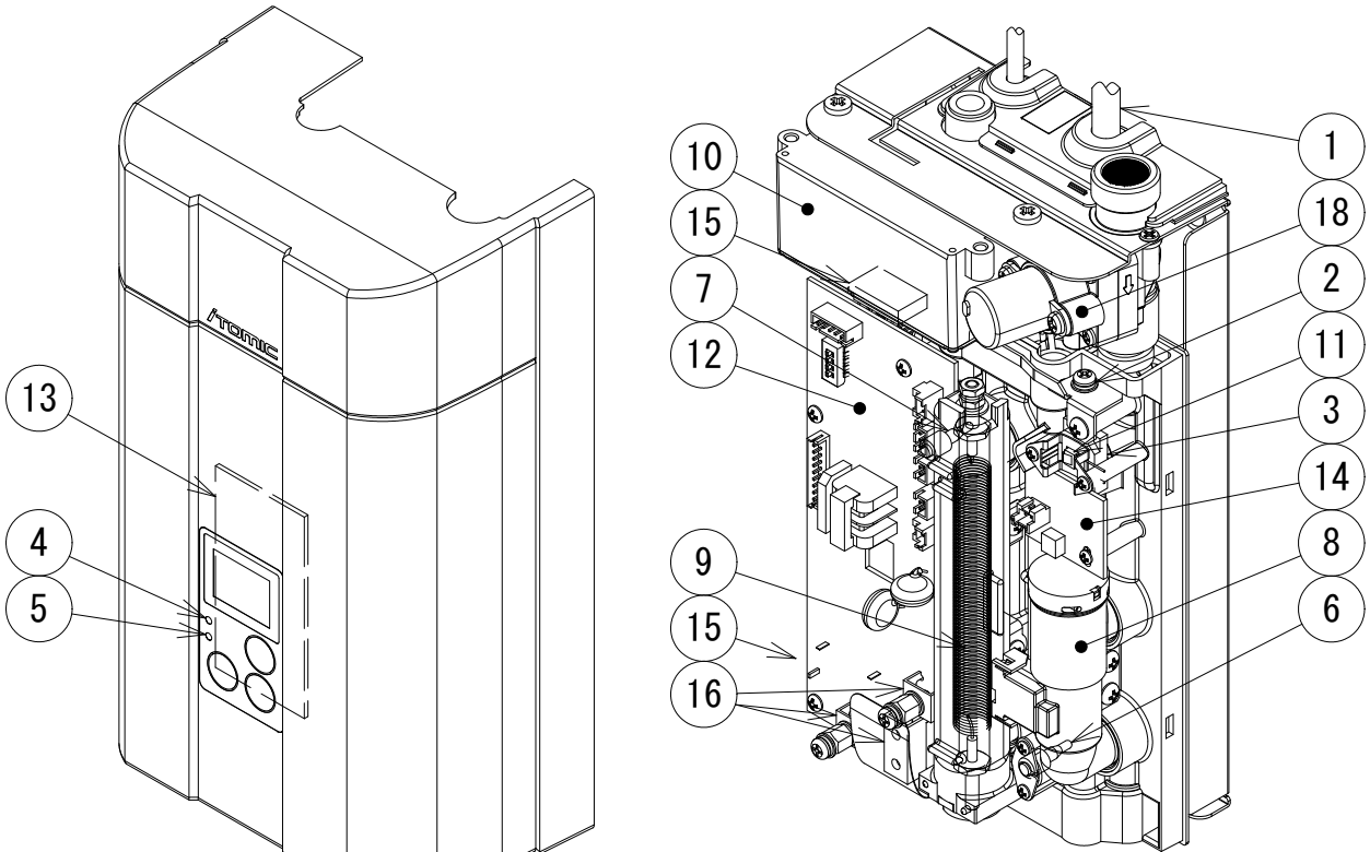
電気部品配置図
