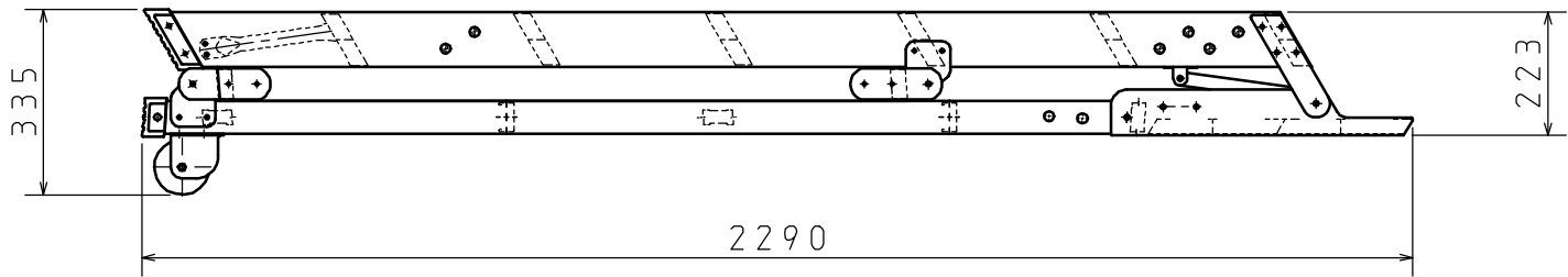
収納状態図
