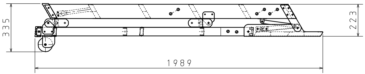
収納状態図
