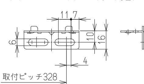
●取付金具下詳細図(S=1:2)
