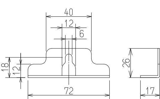
●取付金具上詳細図(S=1:2)
