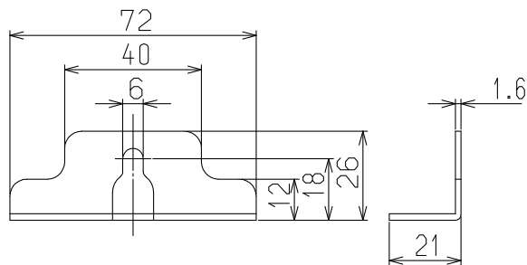
取付金具上詳細 (S=1/2)
