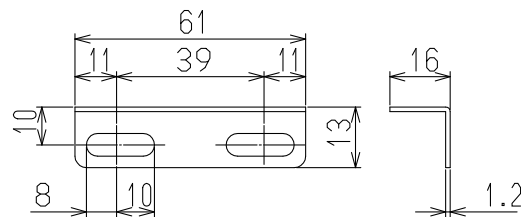
取付金具下詳細 (S=1/2)
